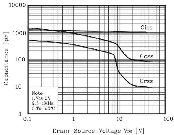
V DS – C T Characteristics
